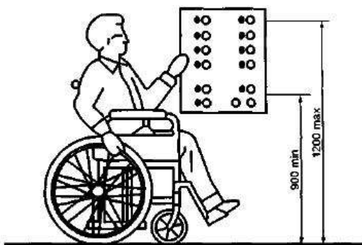
б) Высота органов управления лифтом
