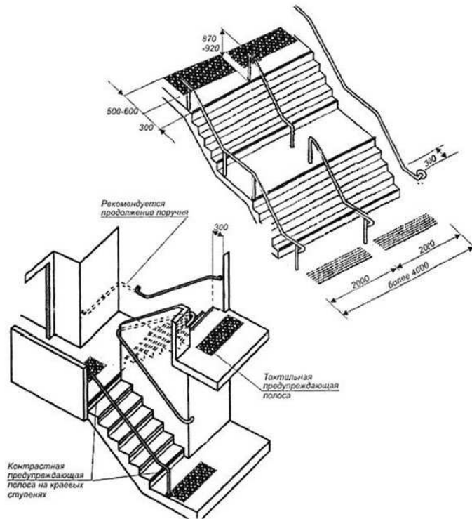
Рисунок В.24 - Параметры лестниц
