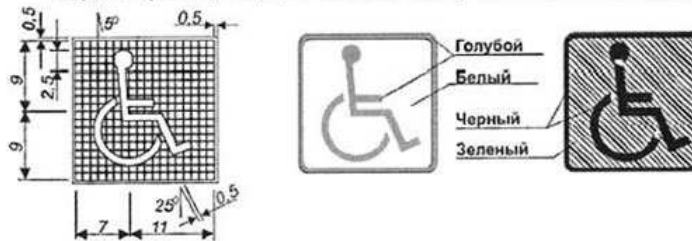
Параметры и пропорции символа доступности для инвалидов
