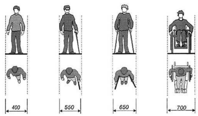
Рисунок В.12 - Параметры зон движения инвалидов
