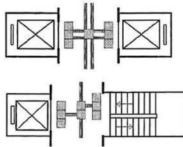
Рисунок Г.18 - Тактильно-контрастные указатели
