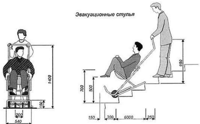
Рисунок В.34 - Автономные транспортные устройства
