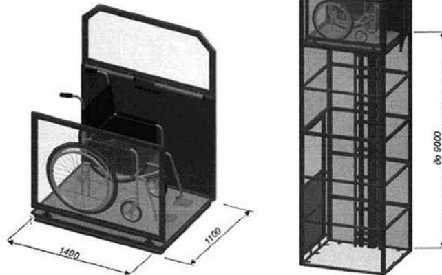
Рисунок В.33 - Параметры вертикальных подъемников
