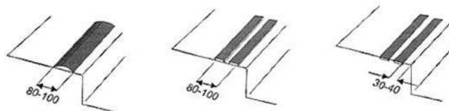
Рисунок В.22 - Предупреждающие контрастные и тактильные полосы
