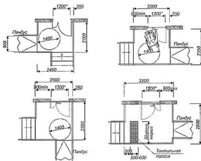
Рисунок В.19 - Площадки перед входами
