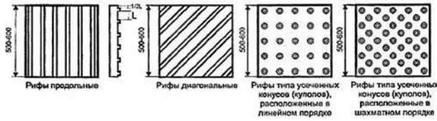
Типы рифления тактильно-контрастных указателей для технологии холодного пластика
