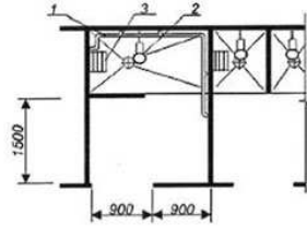
Душевая кабина для инвалида на кресле-коляске
