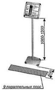
Размещение тактильной полосы перед мнемосхемой
