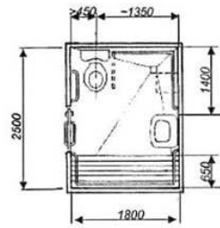
Душевая кабина для инвалида на кресле-коляске
