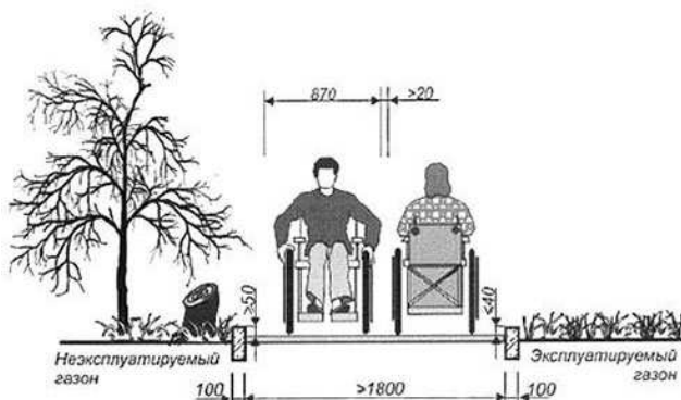
Рисунок В.7 - Организация путей движения на участке
