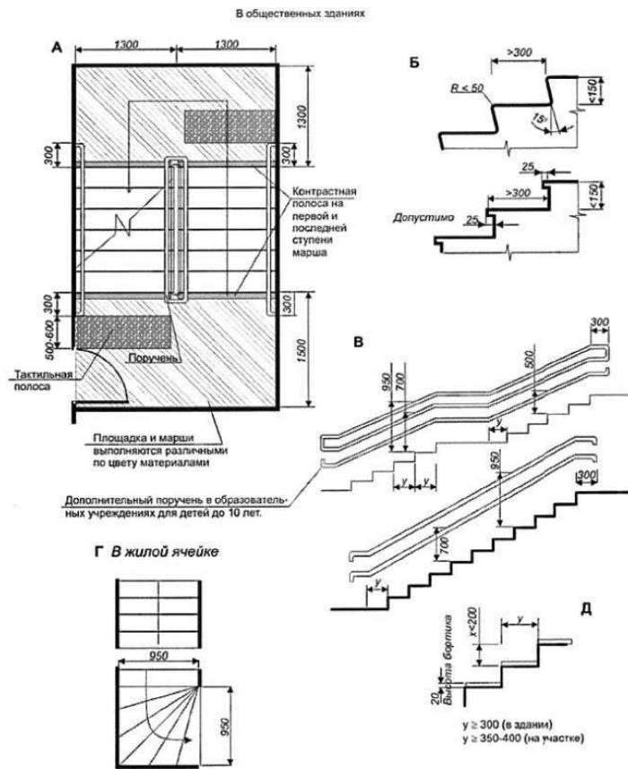
А - минимальные параметры лестничной клетки; Б - максимальные параметры ступени; В - принцип устройства поручня в общественных местах; Г - допустимые параметры внутренней лестницы в жилой ячейке; Д - соотношение ширины проступи и высоты подступенка
