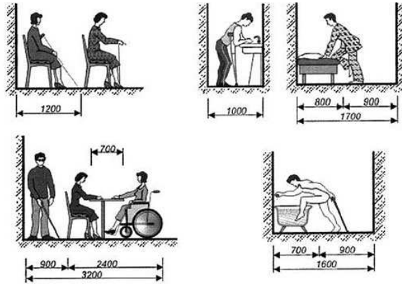
Рисунок Г.4 - Параметры функциональных зон
