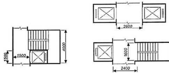
Рисунок В.30 - Габариты лифтов
