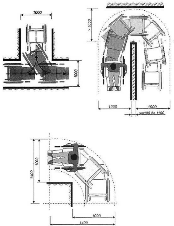
Рисунок В.13 - Размеры поворота и разворота кресла-коляски
