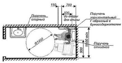
Рисунок Г.12 - Примеры оборудования совмещенного санитарного узла
