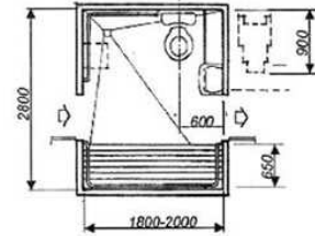
Душевая кабина для инвалида на кресле-коляске
