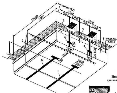
Размещение закладных устройств и разметка ванны для спортивного плавания
