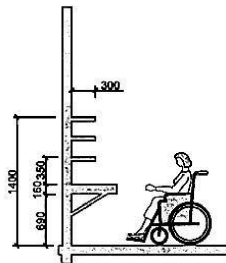
ГАБАРИТЫ УСТАНОВКИ ОБОРУДОВАНИЯ
