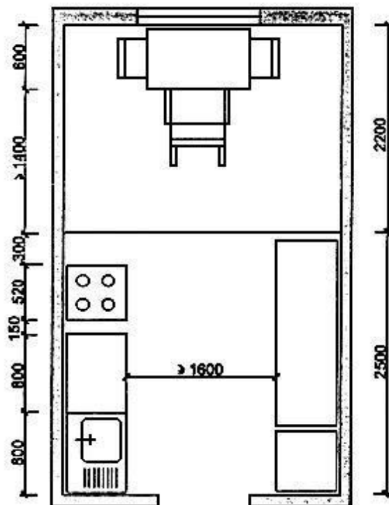
ГАБАРИТЫ УСТАНОВКИ ОБОРУДОВАНИЯ
