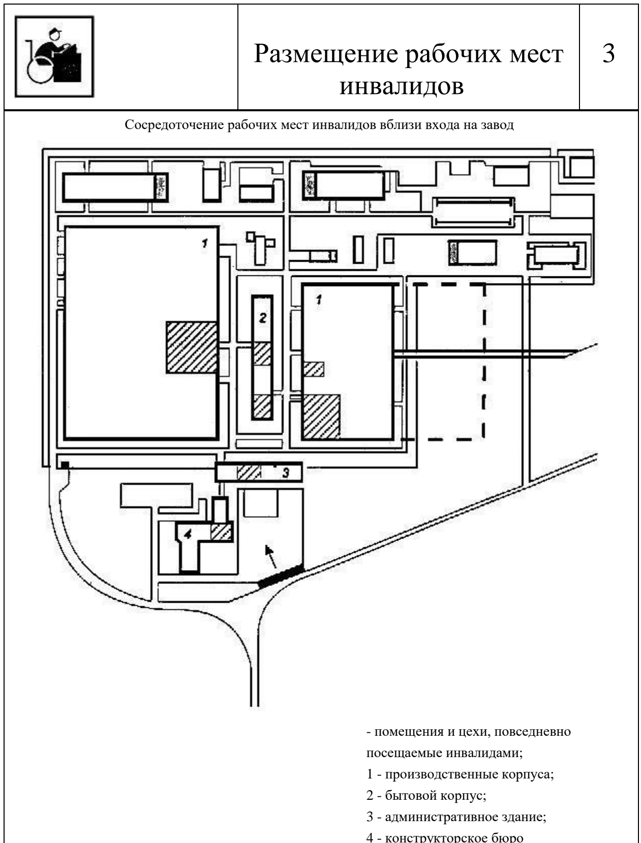
Рис.3. Размещение рабочих мест инвалидов
