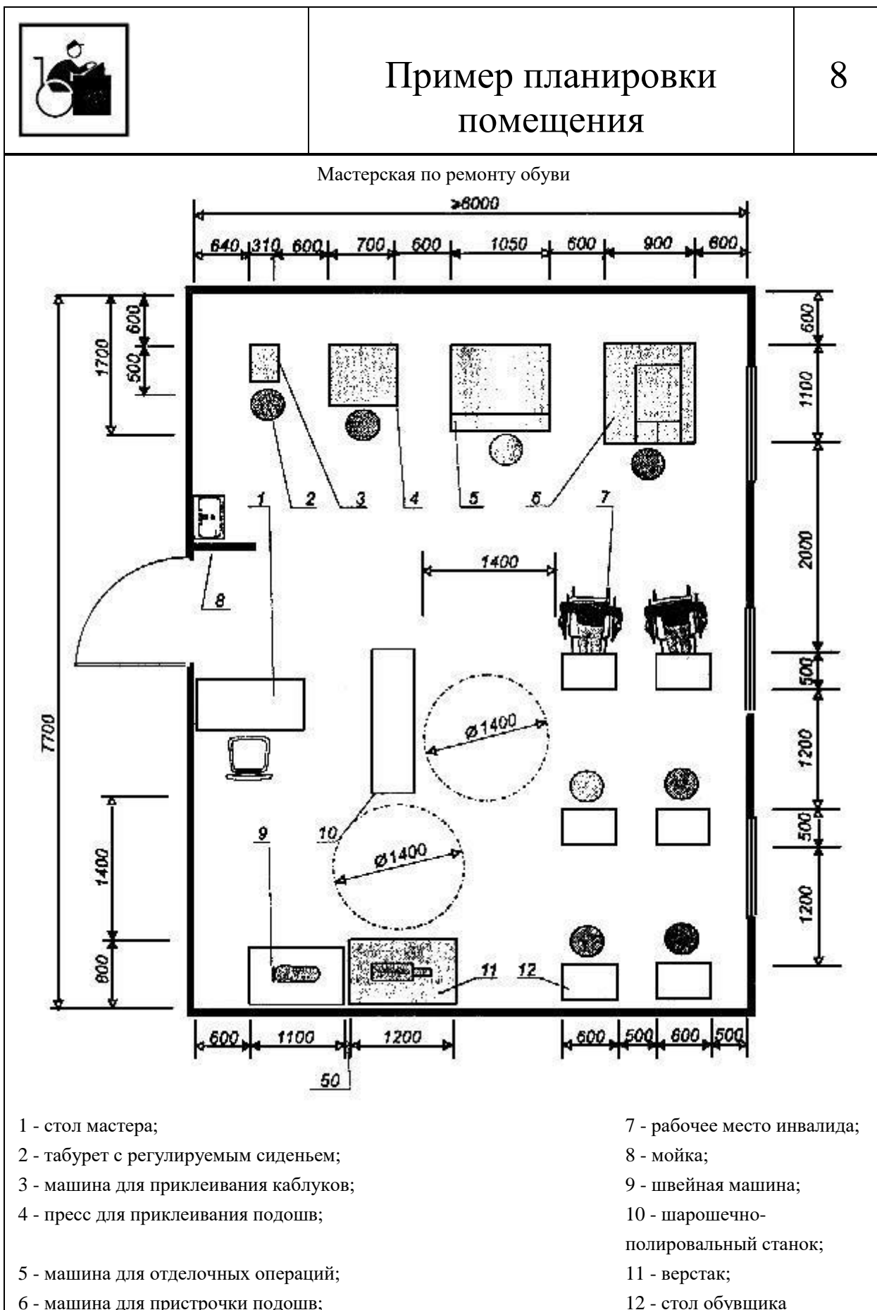
Рис.8. Пример планировки помещения
