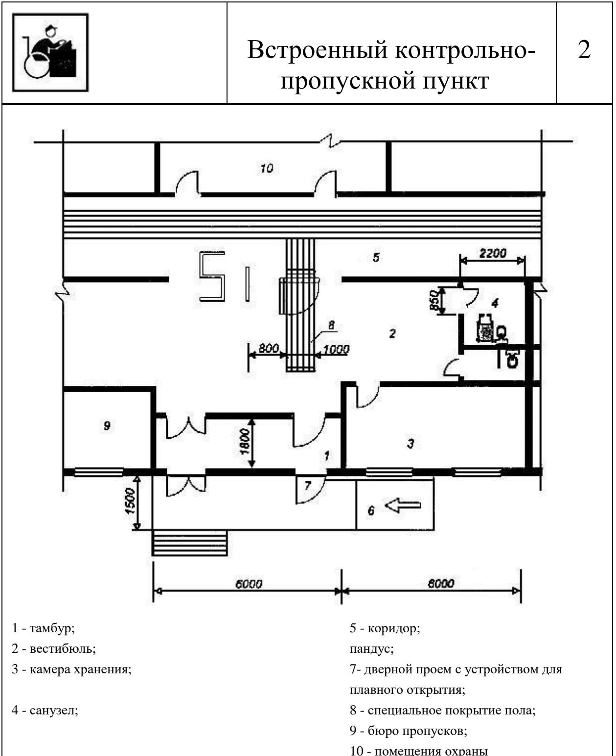
Рис.2. Встроенный контрольно-пропускной пункт
