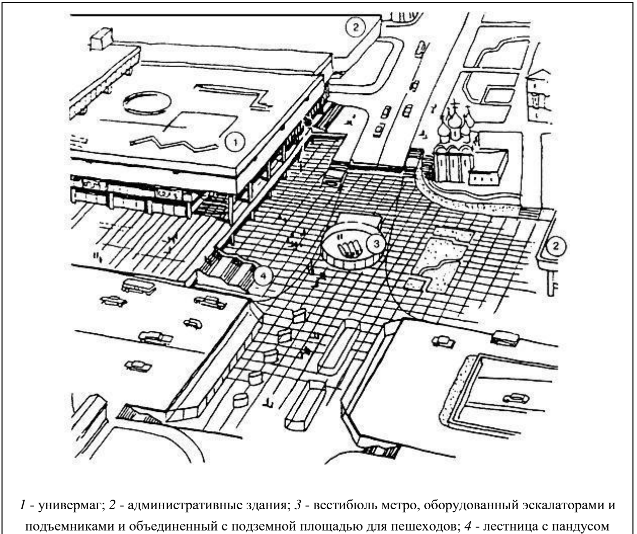
Рис.20 Организация движения транспорта и пешеходов на привокзальной площади
