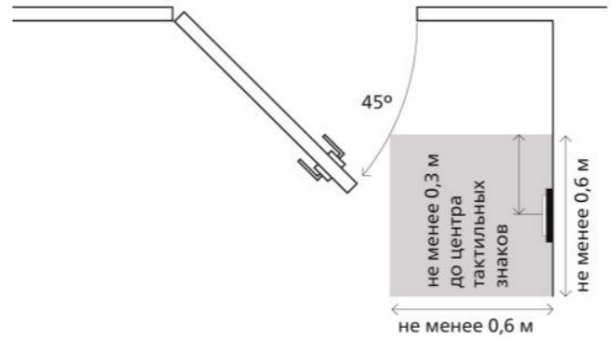
Рисунок 12 — Размещение информации при угловом расположении двери на расстоянии не менее 0,6 м от боковой стены
