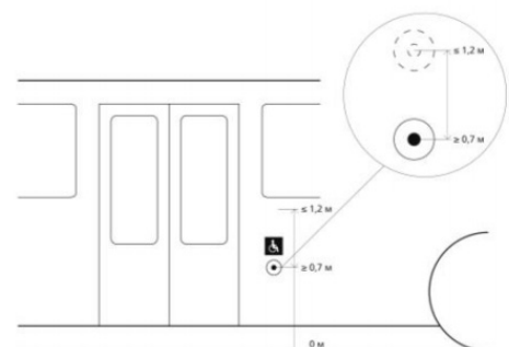
Рисунок 39 — Расположение кнопок персонала на поручнях транспортных средств вызова персонала на внешней стороне кузова транспортных средств
