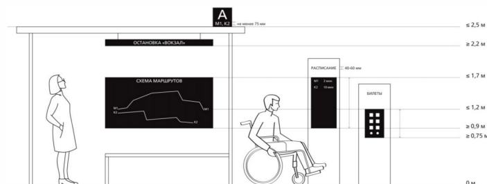
Рисунок 29 — Параметры размещения средств информации на остановочных пунктах
