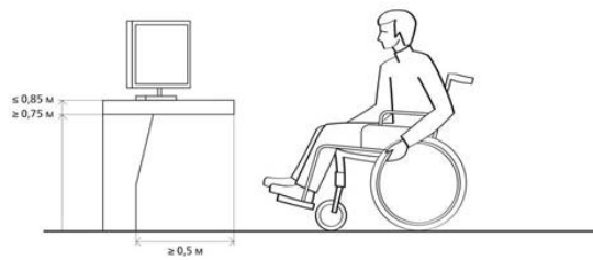
Рисунок Б.6 — Высота рабочей поверхности для обслуживания инвалида, использующего для передвижения кресло-коляску
