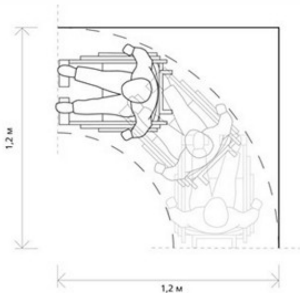
Рисунок Б.2 — Пространство для поворота на 90°
