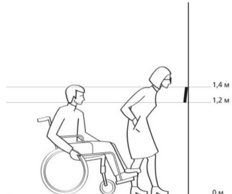
Рисунок 14 — Размещение информации под наклоном для инвалида, использующего для передвижения кресло-коляску
