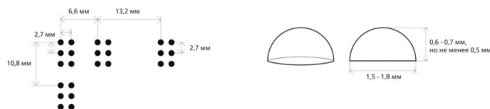
Рисунок 31 — Размеры рельефно-точечного шрифта Брайля
