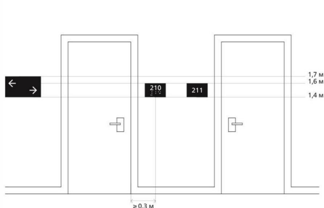
Рисунок 6 — Визуальная информация для идентификации помещений
