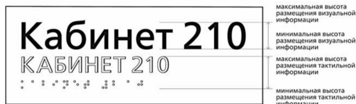
Рисунок 5 — Оси минимальной и максимальной высот размещения визуальной и тактильной информации
